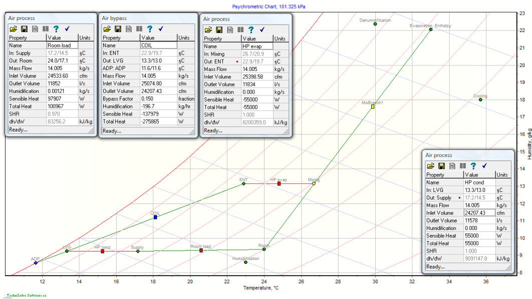
รูปที่ 5. แผนภูมิไซโครเมตริกเครื่องเป่าลมเย็นที่ใช้ฮีทไปป์ช่วยควบคุมอุณหภูมิและความชื้นสัมพัทธ์ ที่อากาศภายนอกสูงสุด
