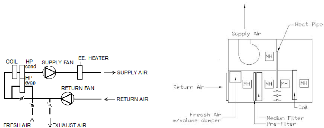
รูปที่ 4. เครื่องเป่าลมเย็นควบคุมอุณหภูมิและความชื้นสัมพัทธ์ที่ติดตั้งฮีทไปป์ช่วยลดการทำงานของฮีทเตอร์ไฟฟ้า
